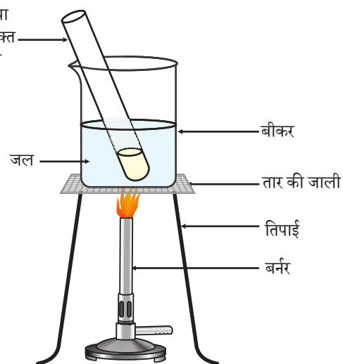
चित्र 4. एस्टर का निर्माण
